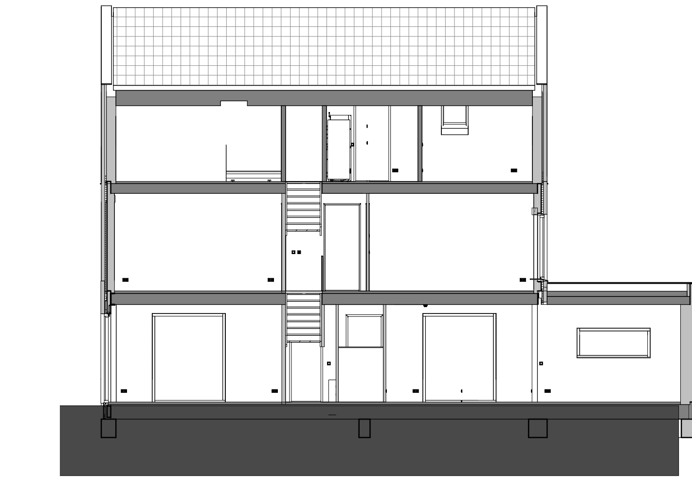
Doorsnede A-A 1:100
