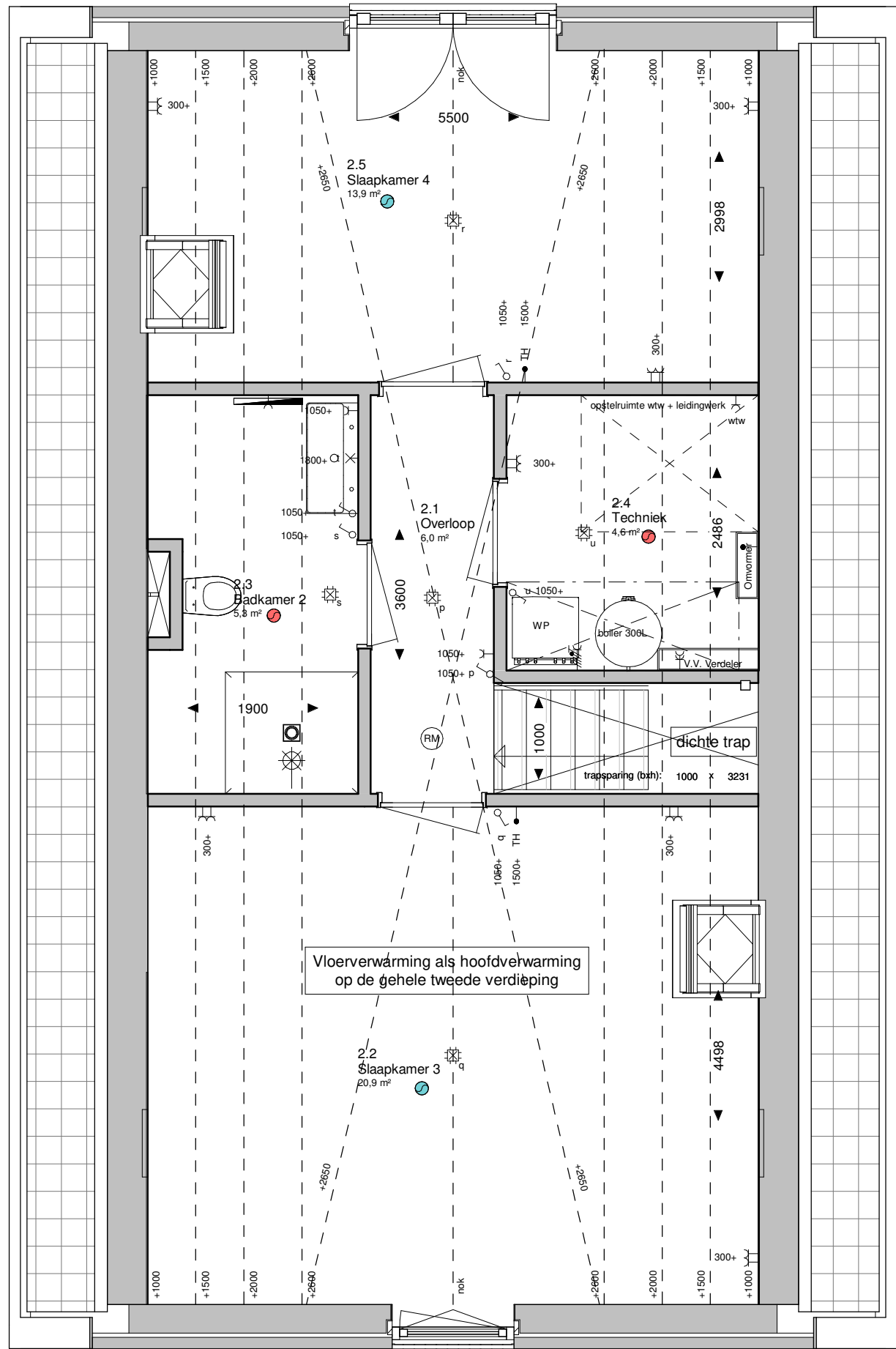
Tweede verdieping 1:50
