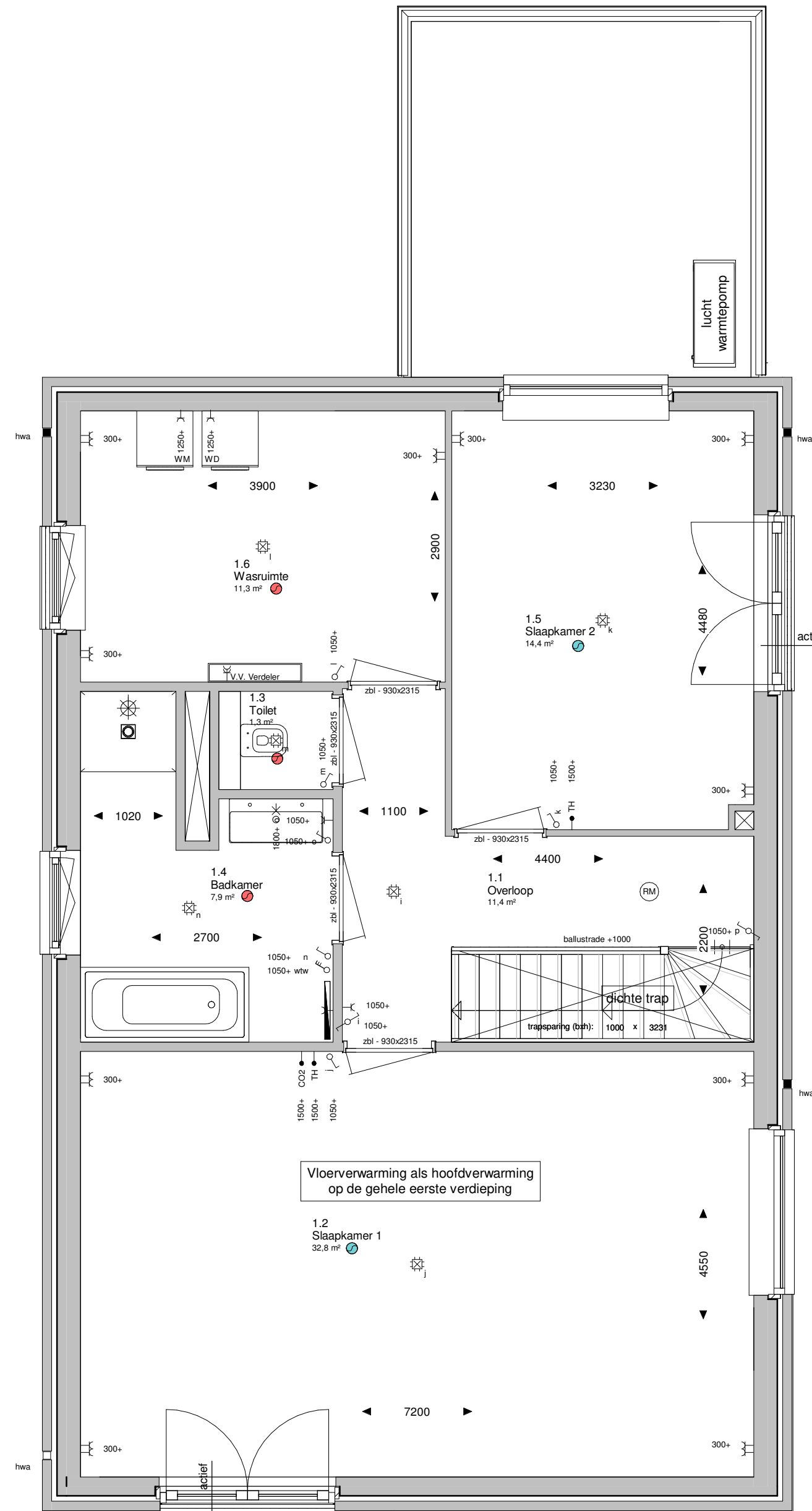
Eerste verdieping 1:50
