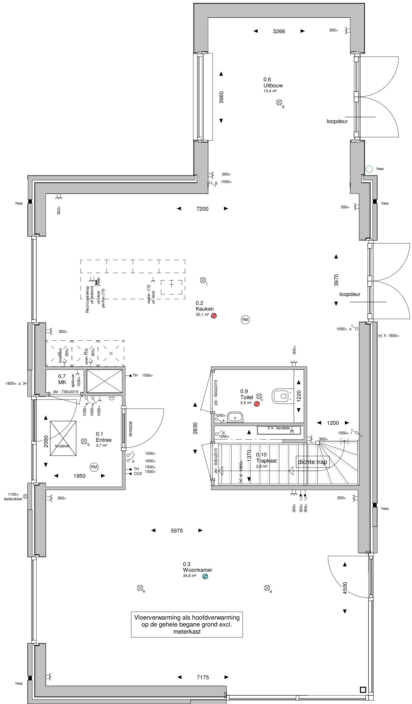
Begane grond 1:50
